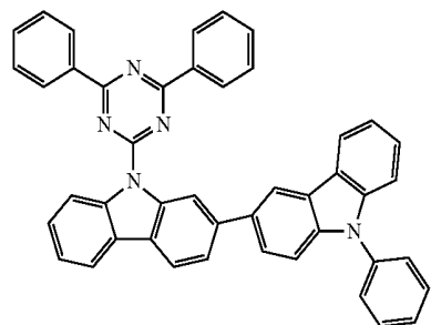
[Formula 48]
