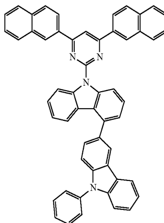
[Formula 58]
