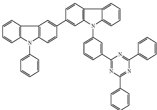
[Formula 260]
