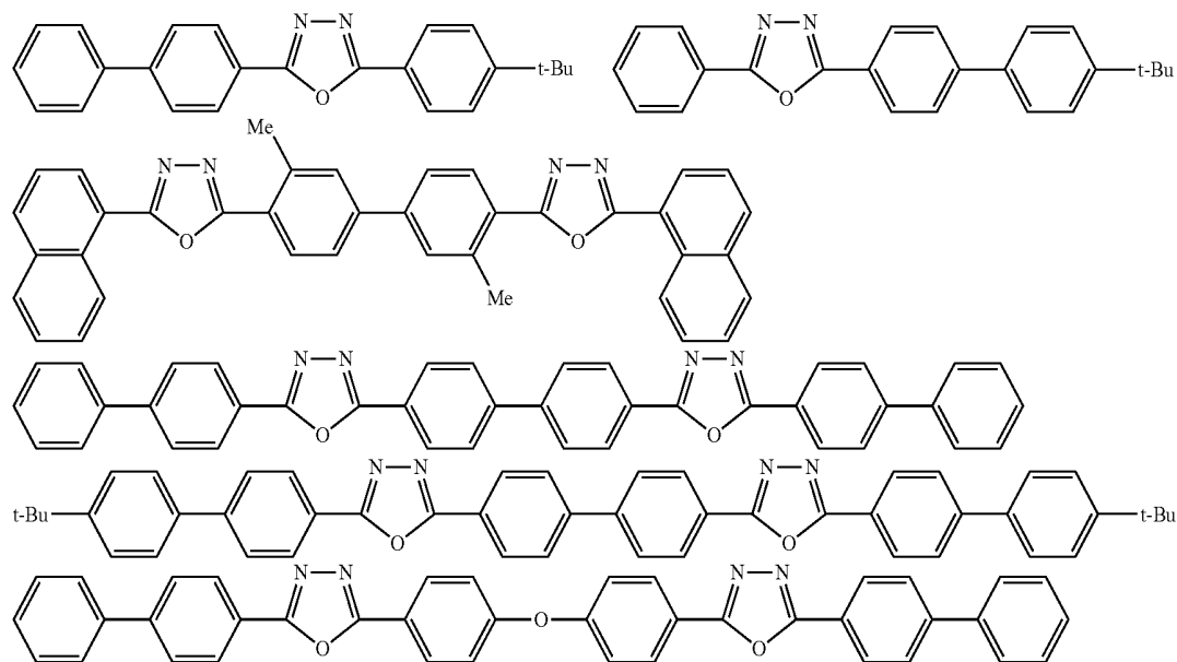
[Formula 243]
