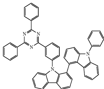
[Formula 71]
