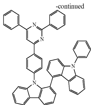
[Formula 71]
