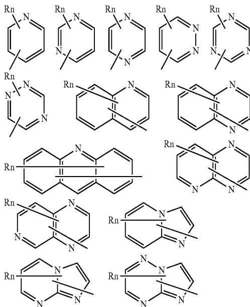
[Formula 246]
