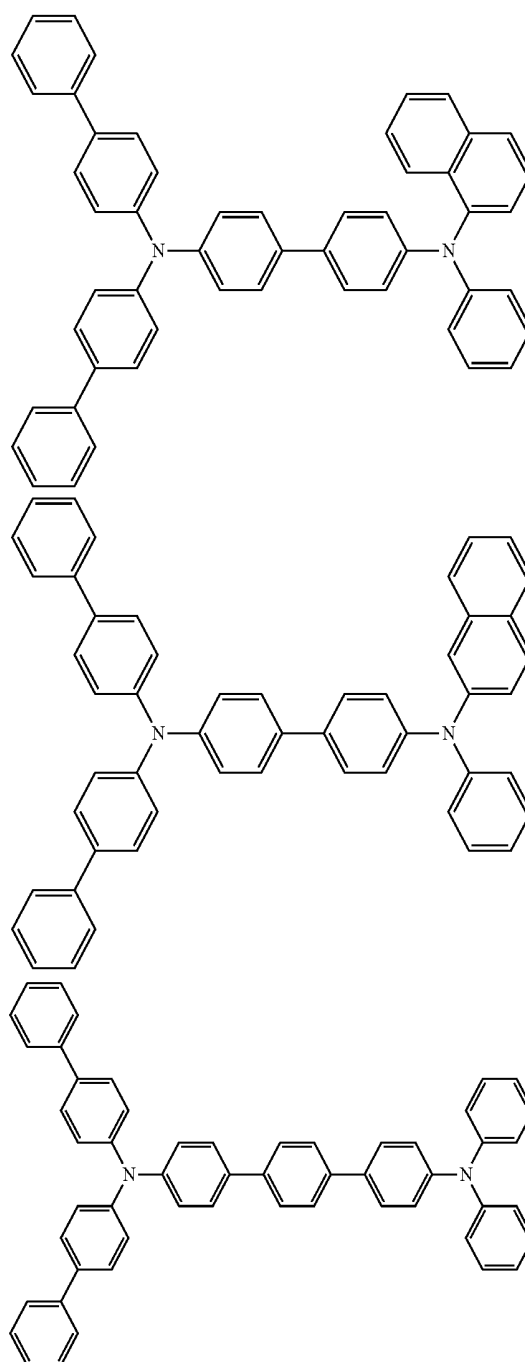
[Formula 236]
